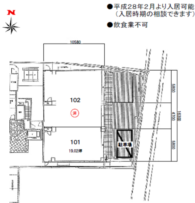
■ 1階平面図
